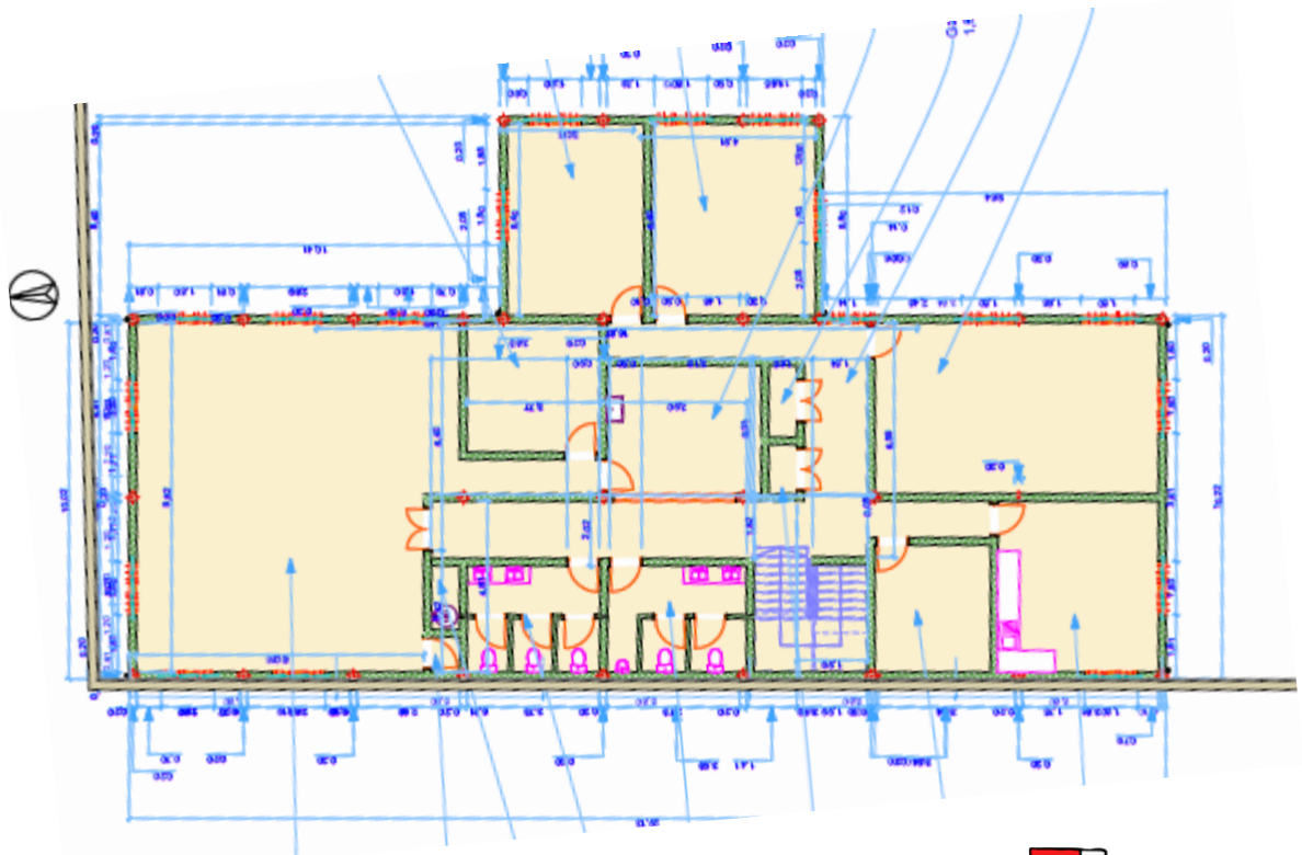
Een ruwe schets van de begane grond van het gebouw
